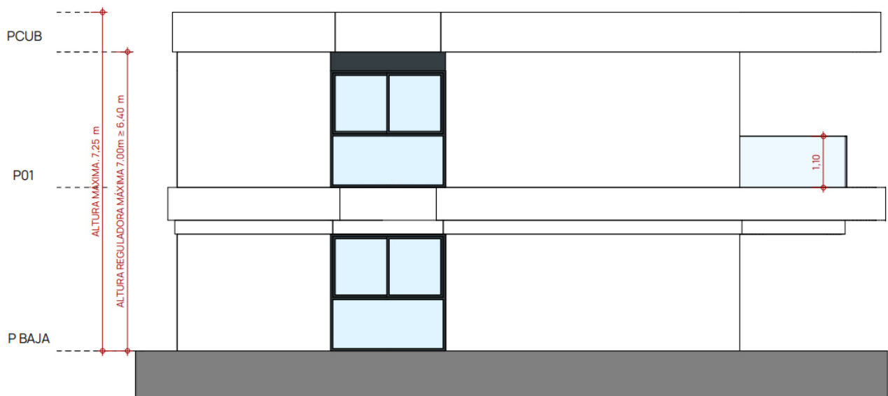
ALZ SUR 1 : 100
